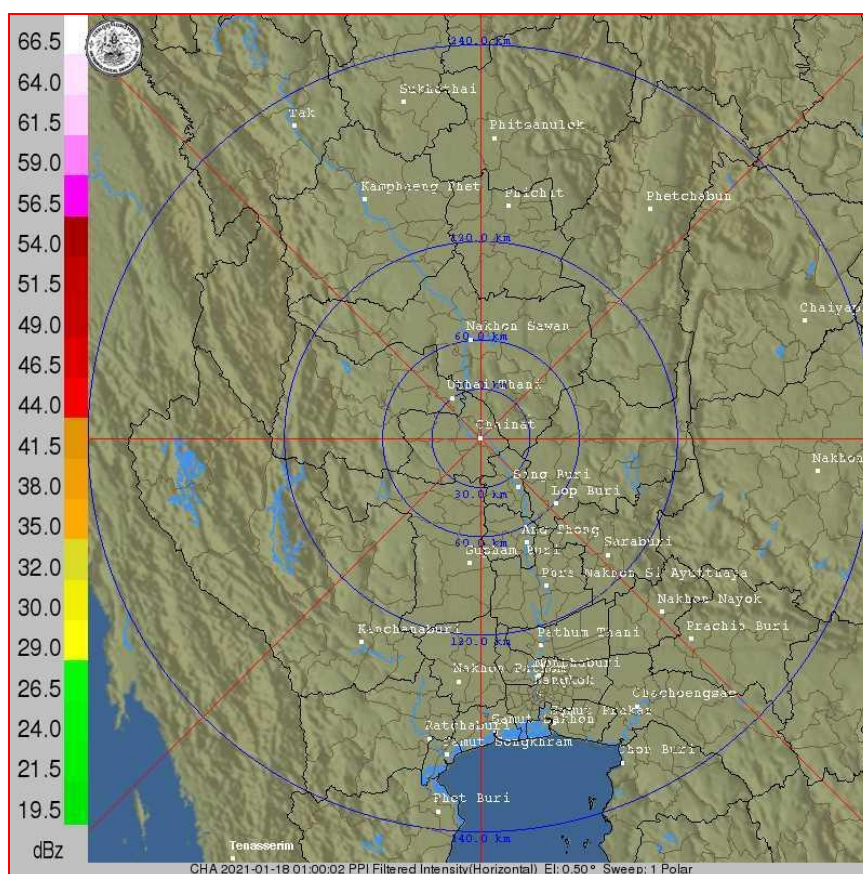
ภาพเรดาร์ที่ตรวจอากาศ “ชัยนาท” ณ วันที่ 18 มกราคม 2564 เวลา 07.00 น. (ที่มา : กรมอุตุนิยมวิทยา https://weather.tmd.go.th/chn.php )
